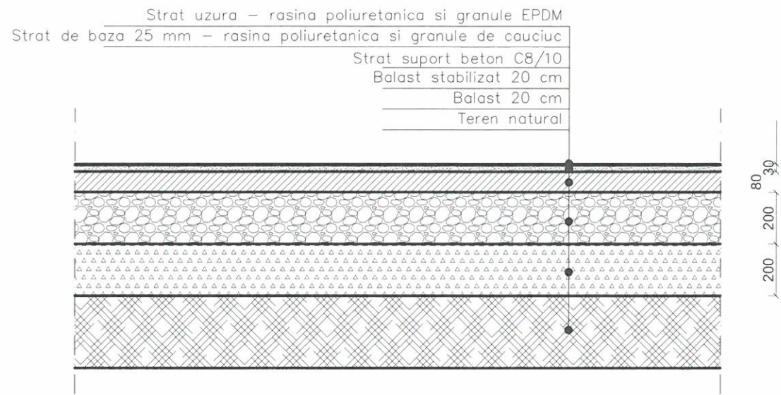
D1: DETALIU – STRATIFICATIE TEREN DE SPORT – SC. 1/20
