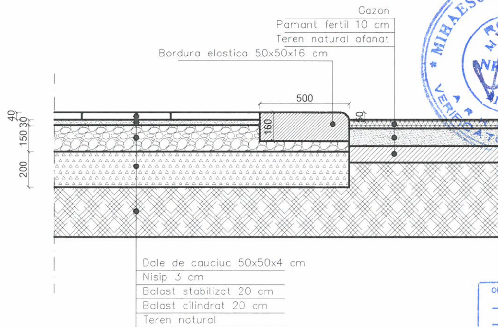
D2: DETALIU – STRATIFICATIE LOC DE JOACA – SC. 1/20
