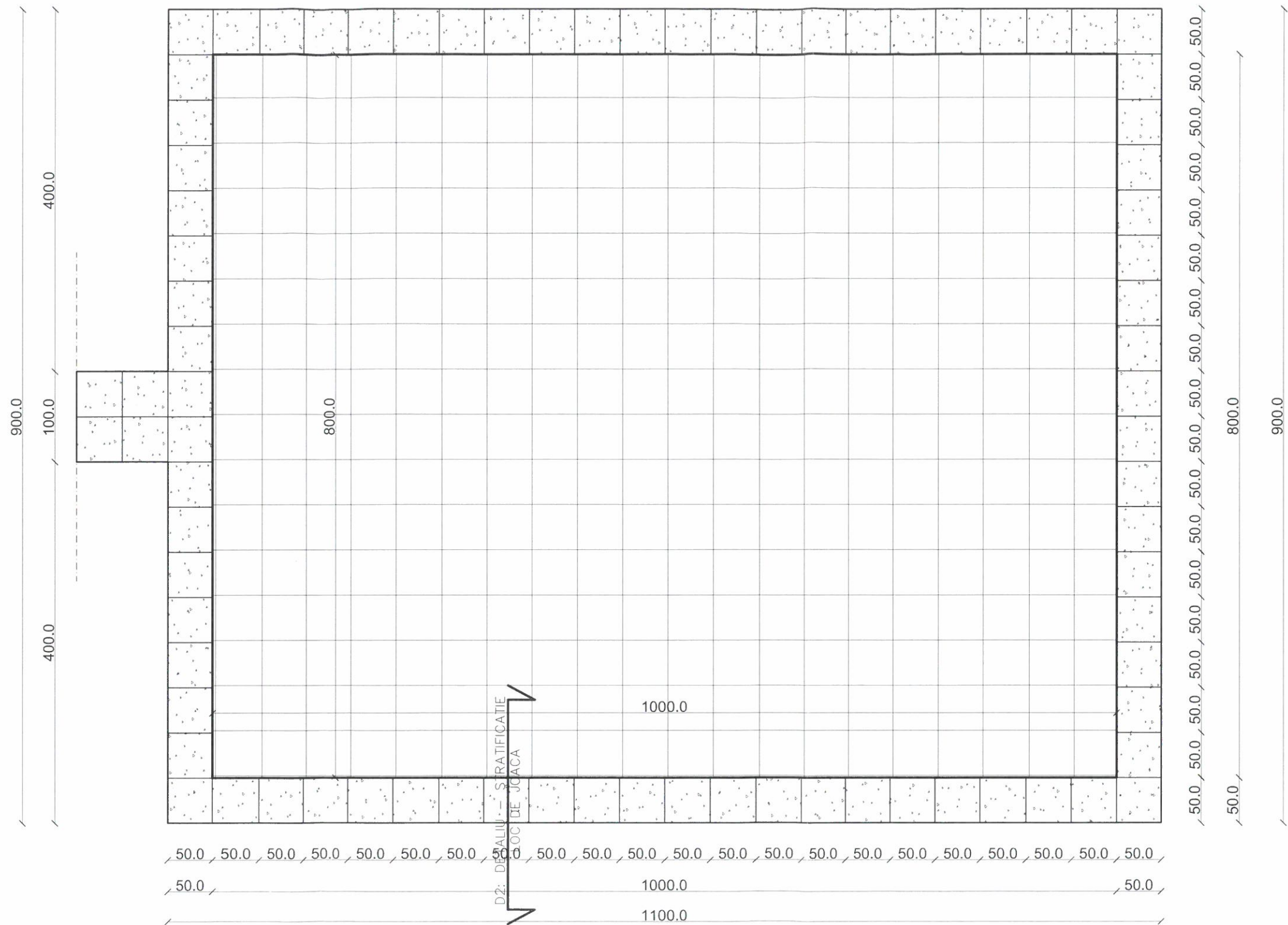
PLAN LOC DE JOACA – SC. 1:50
