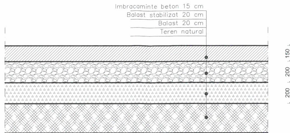
DETALIU – PLATFORMA GOSPODAREASCA – SC. 1/20
